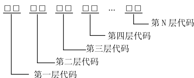
图 1 代码结构图
